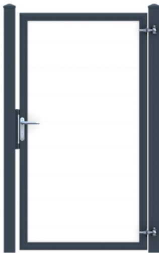
① Öffnungsrichtung nach rechts (Innenansicht)
