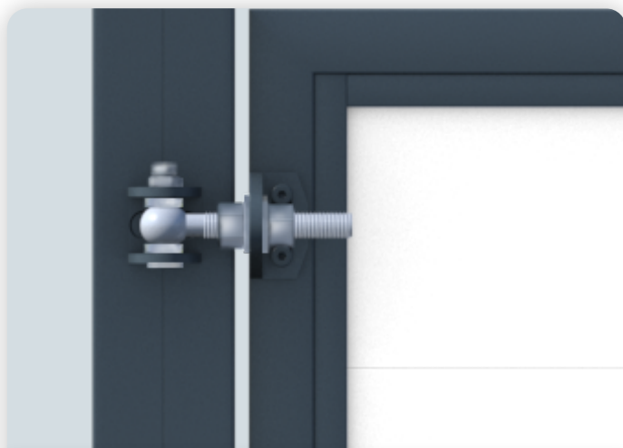
180° Öffnungswinkel M16 Locinox Bänder
